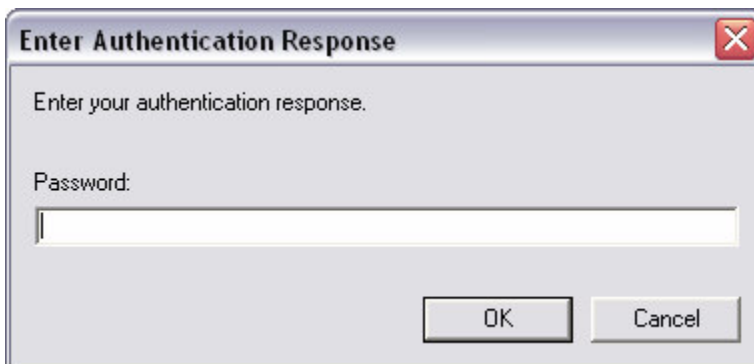
Kuva 4 - Salasana-ikkuna
