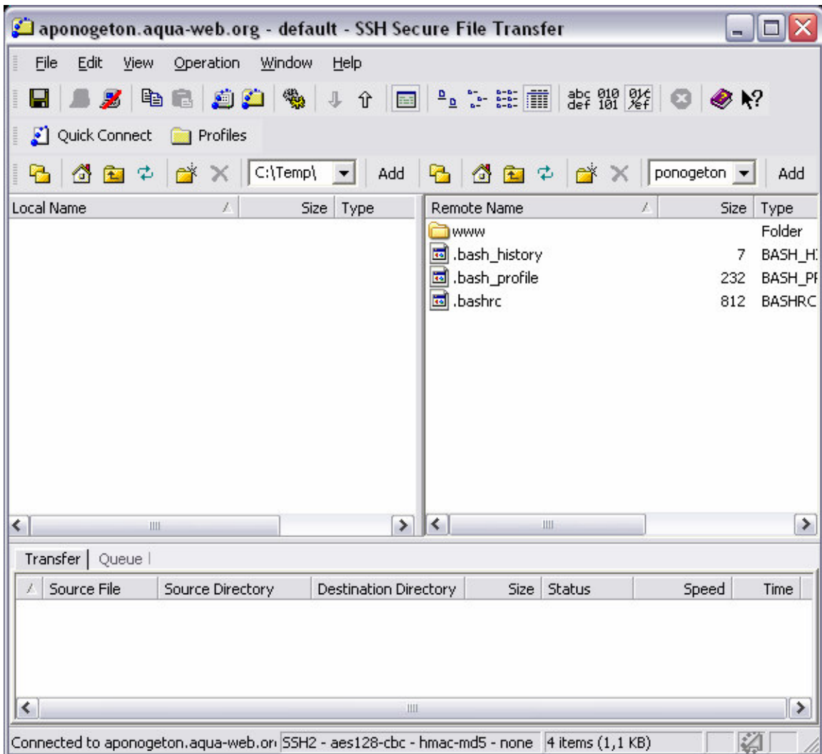
Kuva 6 - Perillä ollaan...
